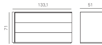
Elemento 3 cassette P=51,2 H=70,4
